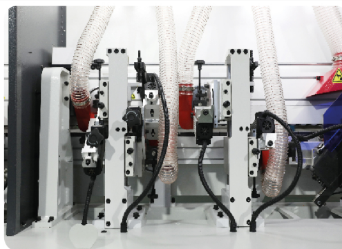
ایستگاههای فرز تخت و ردیوس Trimming
