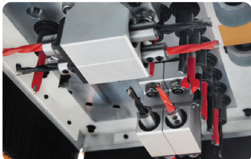
هد سوراخ کاری بالا (دقیق) Precision top drilling head
