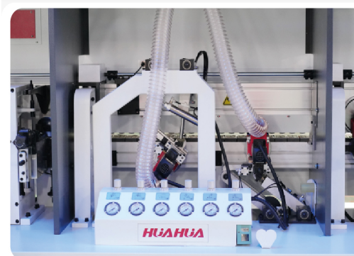
فرز کرنر Corner Rounding
