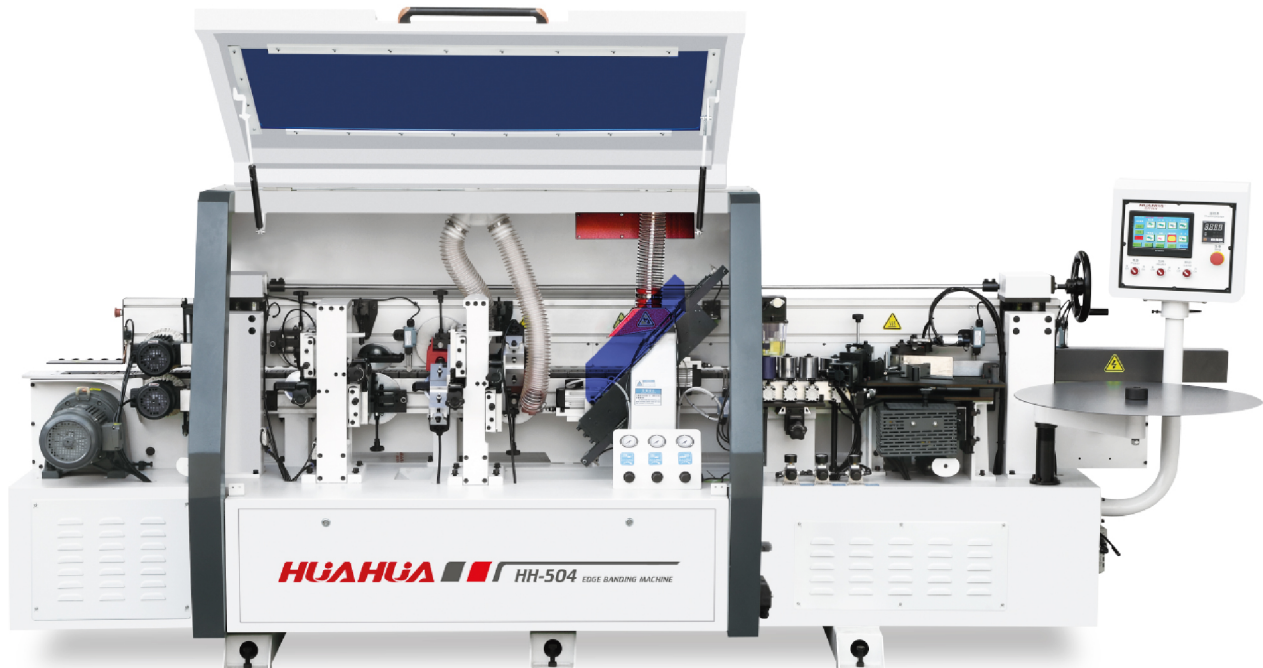
چهار غلطک فشار Four-wheel pressing
