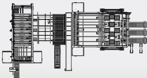
چیدمان دستگاه Layout Plan
